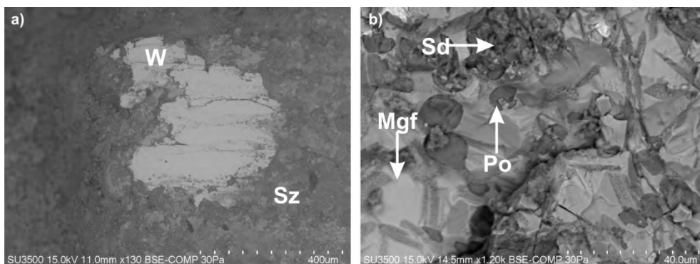
Rys. 4. Obraz SEM żuźła hutniczego: a) szkliwo (Sz) z wydzieloną fazą wustytową (W), b) Mgf - magnesioferyt, Po - portlandyt, Sd - srebrodolskit
