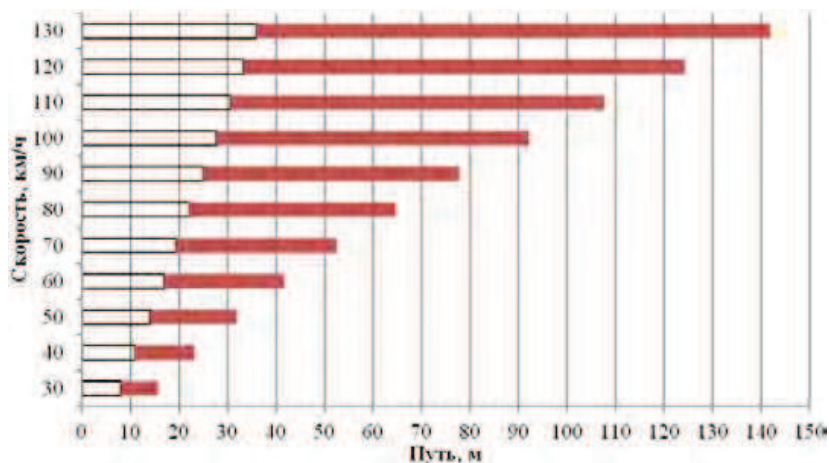
Рис. 2. Тормозные и остановочные пути при экстренном торможении
